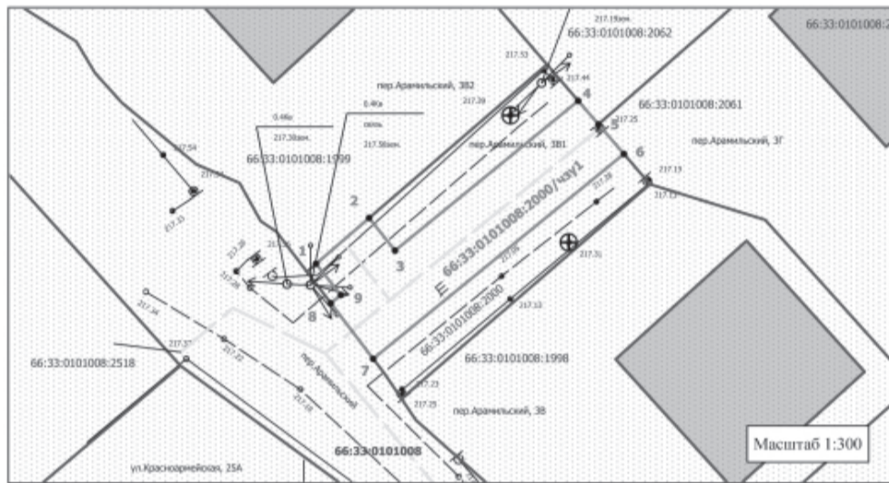
Схема расположения границ публичного сервитута на часть земельного участка с кадастровым номером 66:33:0101008:2000 для размещения распределительного газопровода низкого давления к жилым домам 3В/2, 3В, 3Г, 3Д пер.Арамилский, г.Арамиль
