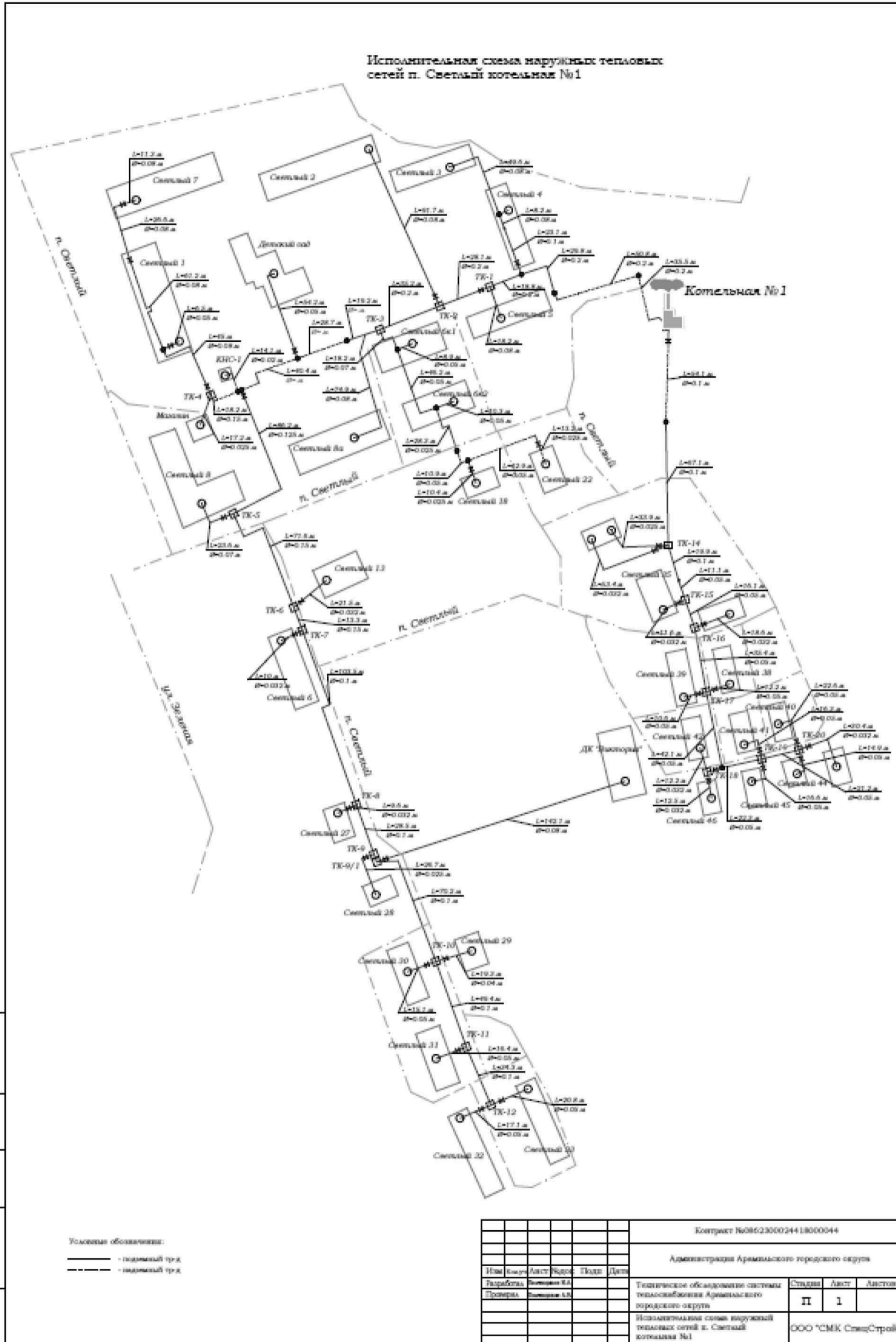
Рис. 5 – Исполнительная схема наружных тепловых сетей котельной №1
